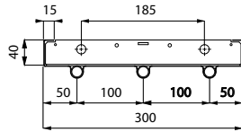
DS-ST18-3-060; 6 Pipes
